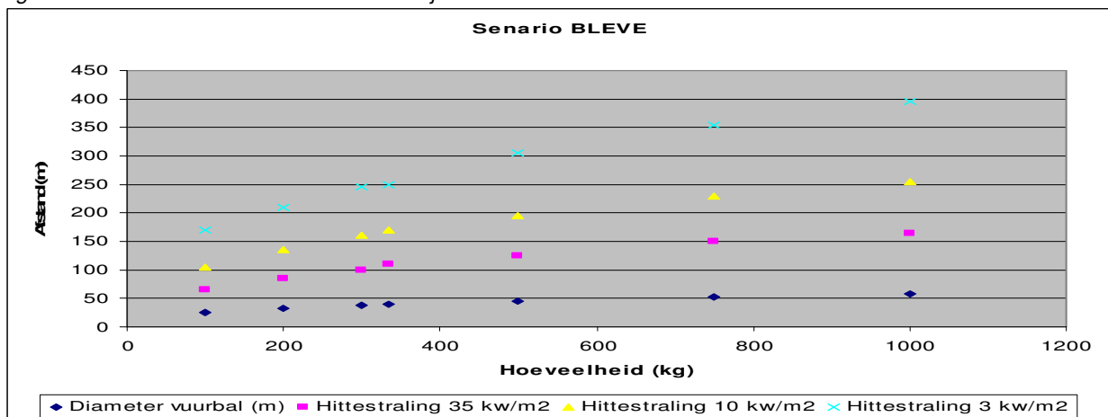
Figuur 5.4.2: minimale afstanden in meters bij het scenario BLEVE
